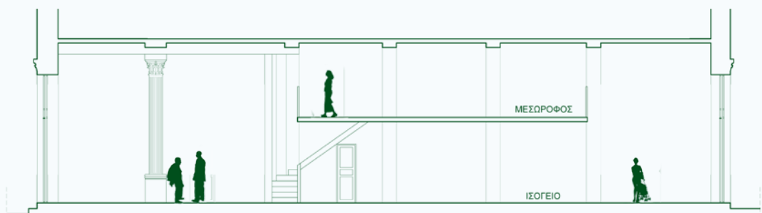
ΧΩΡΟΣ Α, ΥΠΑΡΧΟΥΣΑ ΚΑΤΑΣΤΑΣΗ, ΤΟΜΗ ΚΑΤΑ ΜΗΚΟΣ
